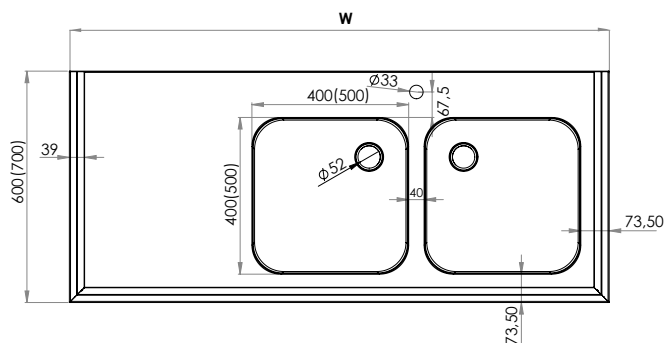
STÓŁ ZE ZLEWEM DWUKOMOROWYM
