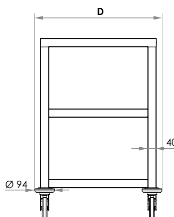
Rzut z przodu
